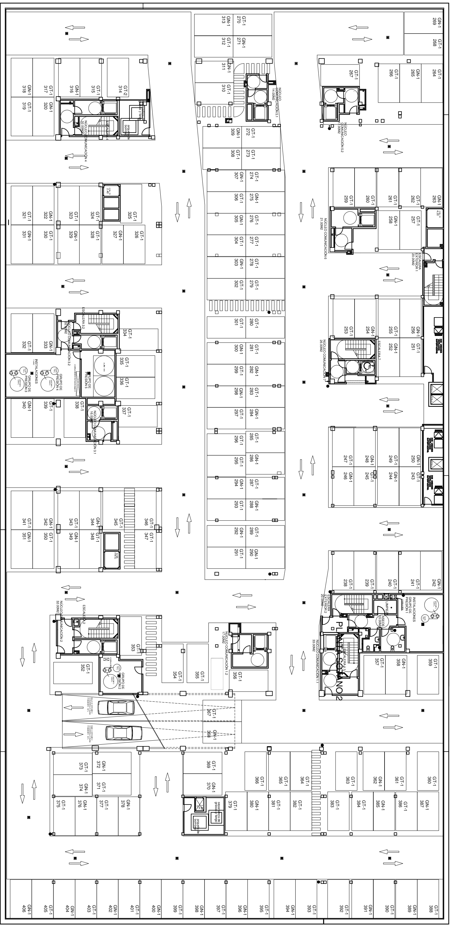
PLANTA SÓTANO 3
